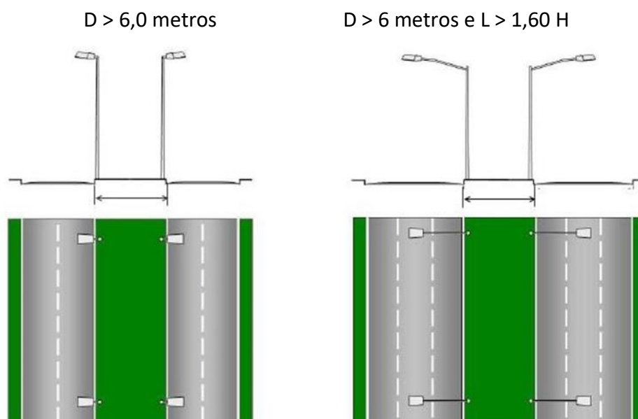
Figura 7: Posteamento central nos canteiros maiores que 6 metros
